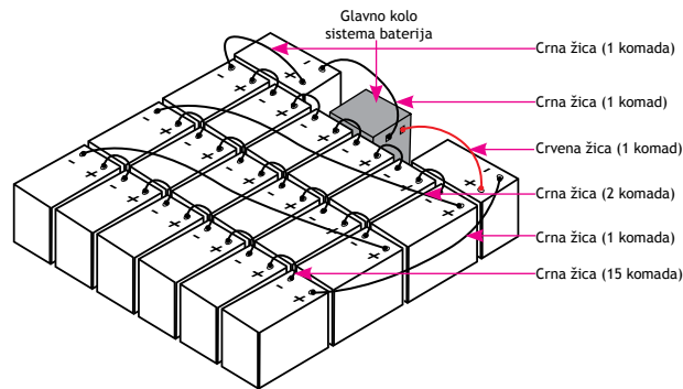
Dijagram povezivanja baterija
