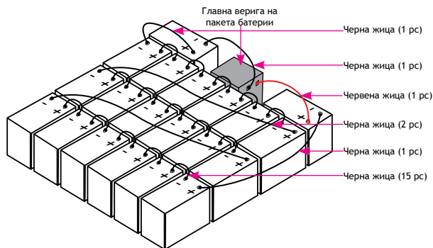
Диаграма на свързване на батериите
