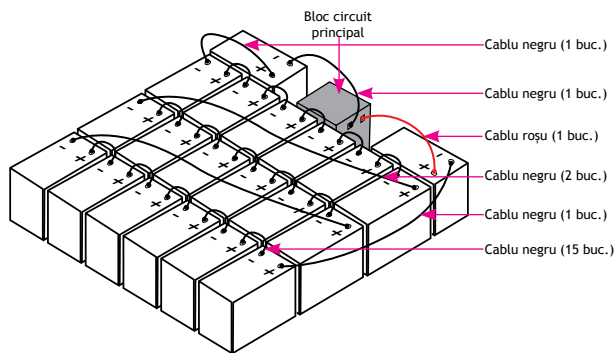
Diagrama de conectare a bateriilor
