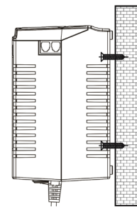
Ábra3. Függőleges felszerelés
